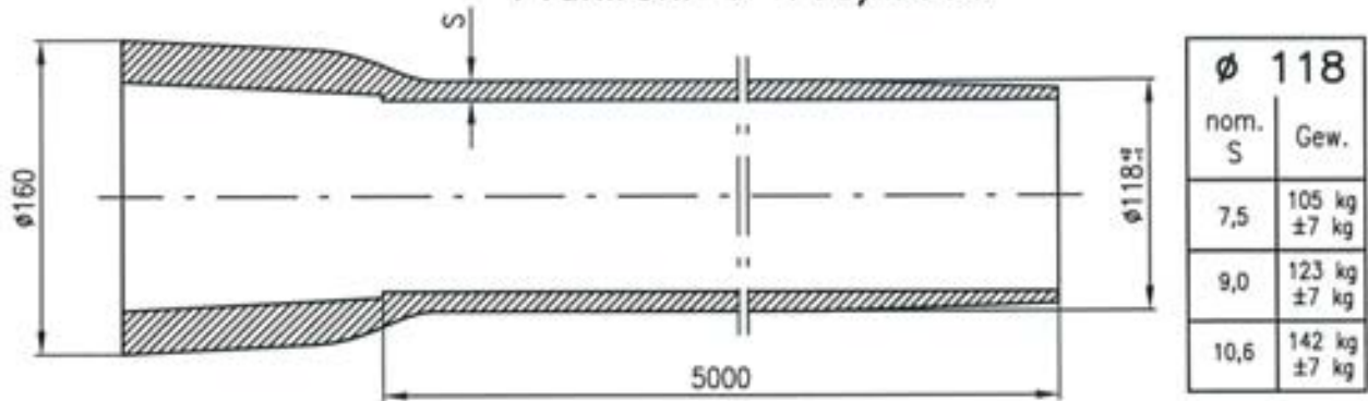
Pfahlrohr \phi 118/5000
