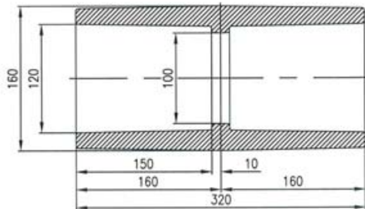
Muffe für Pfähle \varnothing 118
