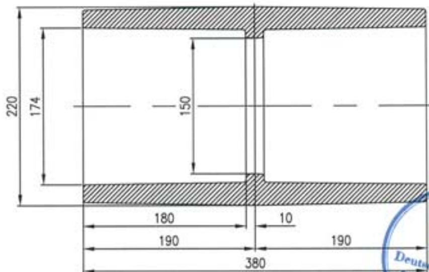
Muffe für Pfähle \varnothing 170
