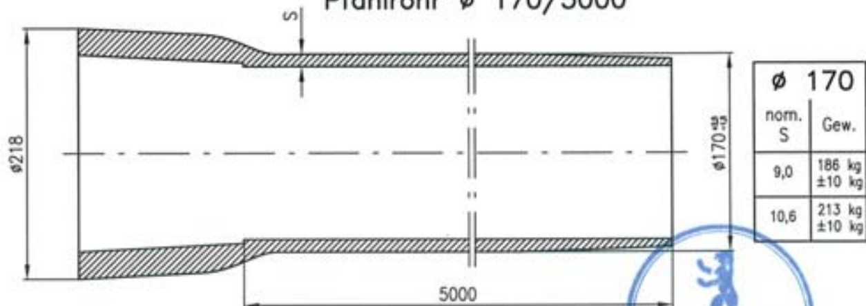
Pfahlrohr \phi 170/5000
